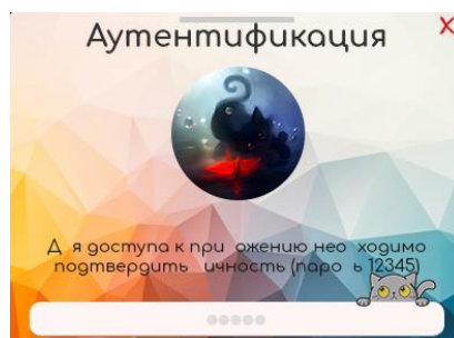
Рисунок 4 – Окно аутентификации
